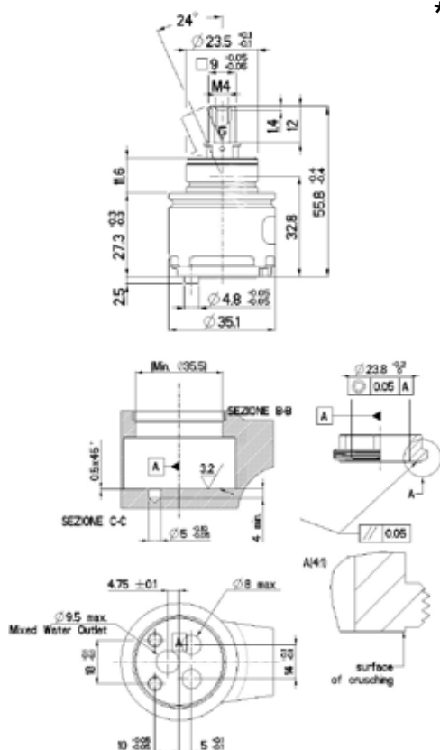
limitatore di portata e temperatura LPT adjustable flow rate and temperature limiter LPT
