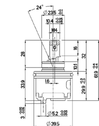
limitatore di portata e temperatura LPT adjustable flow rate and temperature limiter LPT
