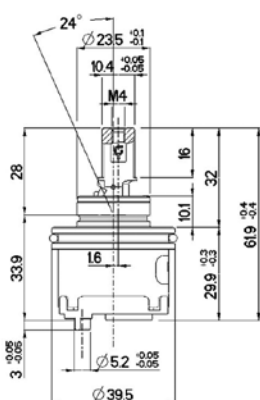
limitatore di portata e temperatura LPT adjustable flow rate and temperature limiter LPT
